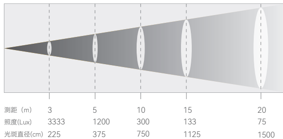
光束角度42°
