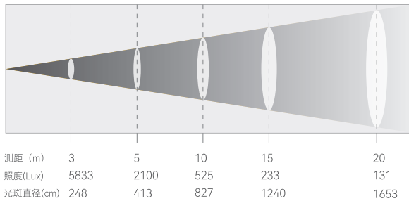
光束角度45°
