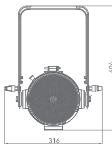
正视图
