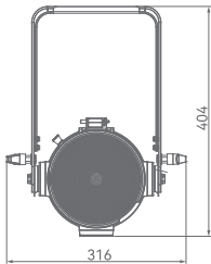
正视图
