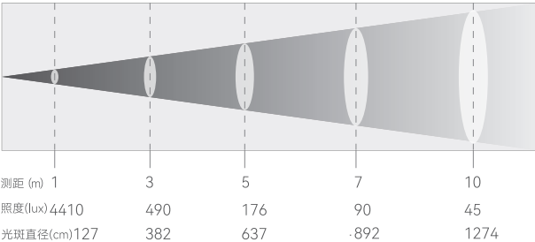
光束角度 65°
