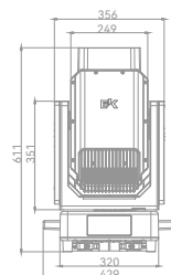
正视图
