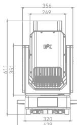
正视图
