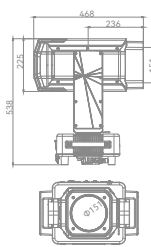
顶视图
