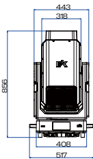
正视图
