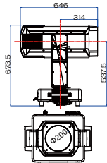
顶视图
