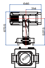
顶视图
