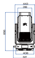
正视图
