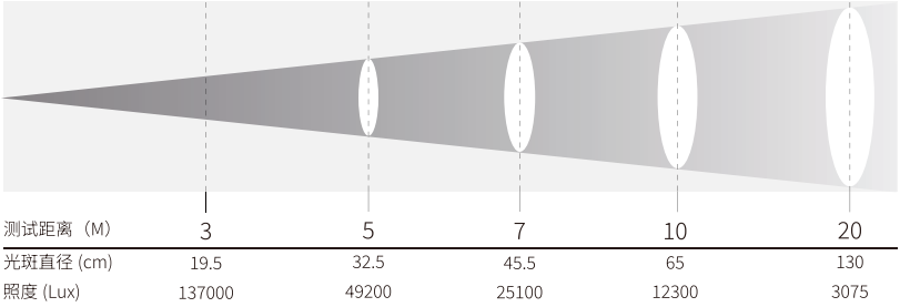
光束角度：6°
