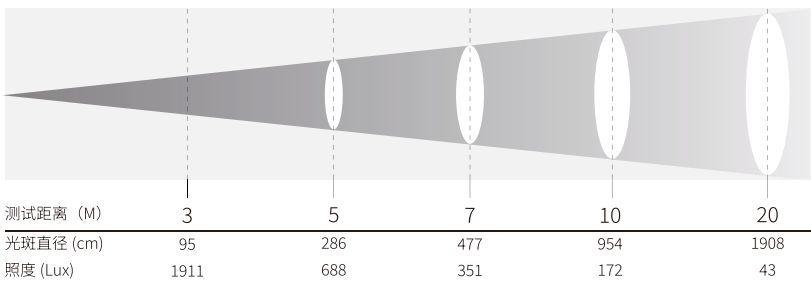
光束角度：51°
