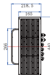
正视图
