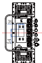
背视图
