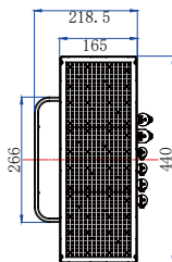
正视图
