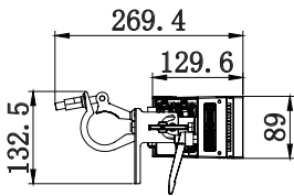
侧视图
