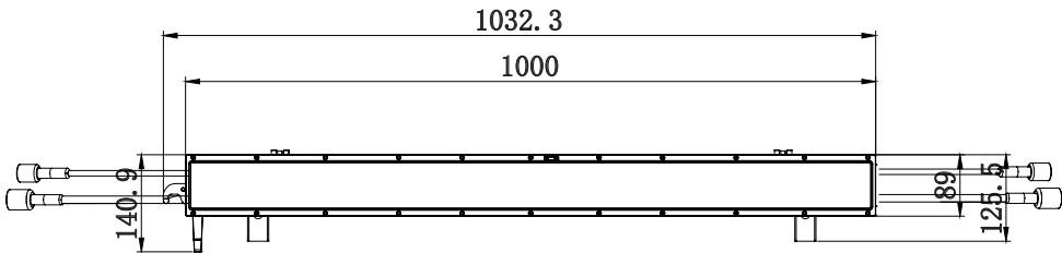
正视图
